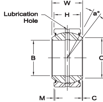
GEZ..ES-2RS SEALED
